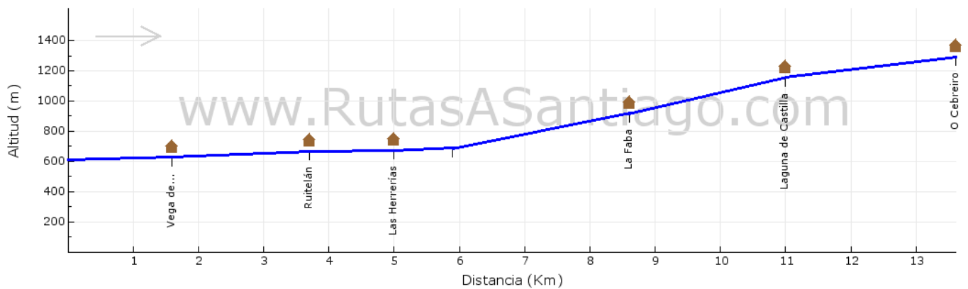
PERFIL Altitud vs. Distancia (Ambasmestas-O Cebreiro)
